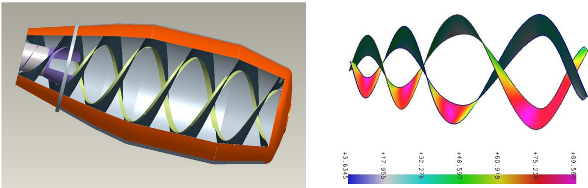
双对数变螺距 3D 设计
